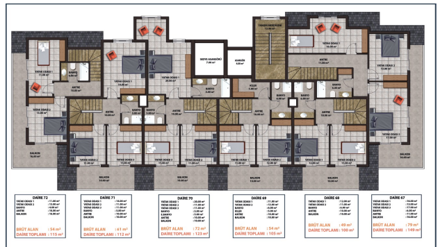
B BLOK ÇATI KATI PLANI
