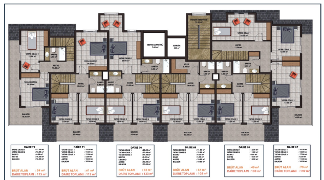
B BLOK ÇATI KATI PLANI
