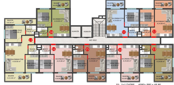
F BLOK / BİRİNCİ KAT PLANI
