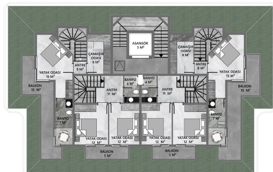
B BLOK ÇATI KATI PLANI
