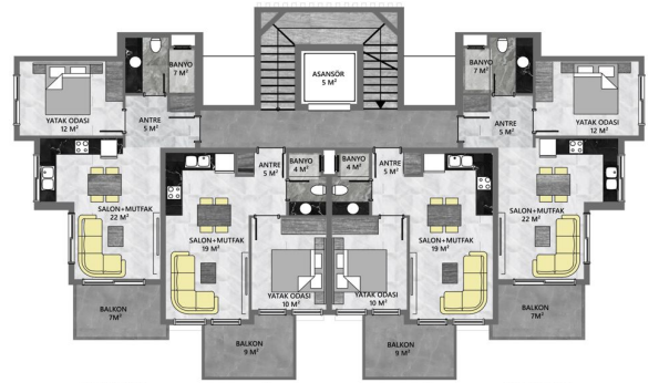
B BLOK 1.KAT PLANI
