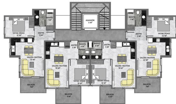
8 NOLU DAİRE BRÜT: 61 M 2 NET: 53 M 2 7 NOLU DAİRE BRÜT: 55 M 2 NET: 47 M 2 6 NOLU DAİRE BRÜT: 55 M 2 NET: 47 M 2 5 NOLU DAİRE BRÜT: 61 M 2 NET: 53 M 2
