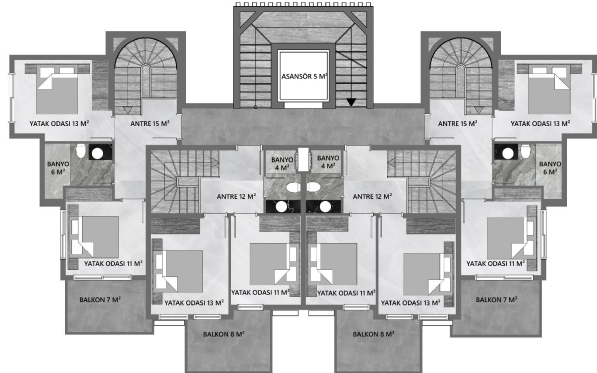
B BLOK ZEMİN KAT PLANI
