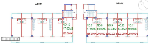
1. KAT PLANI ÖLÇEK : 1/200
