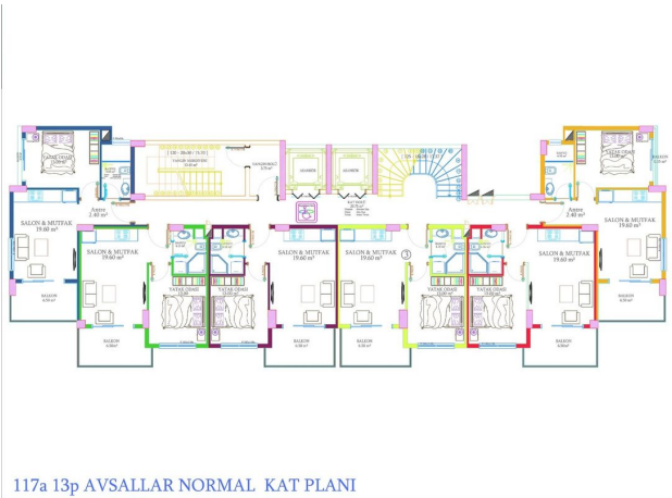
117a 13p AVSALLAR NORMAL KAT PLANI
