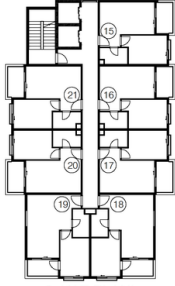
3. KAT PLANI
