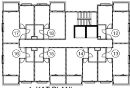
1. KAT PLANI
