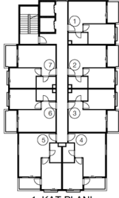
1. KAT PLANI
