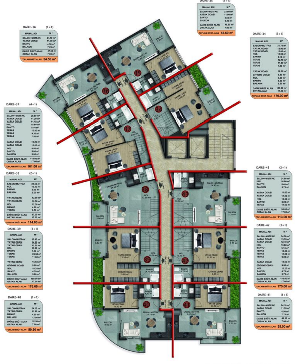
B BLOK 3. KAT PLANI
