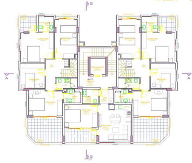
A-D-E BLOK ZEMİN PLANI (+1.50 KOTU)
