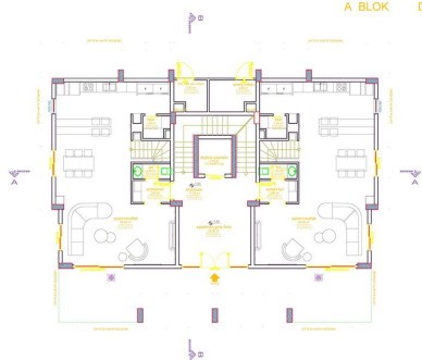
A-D-E BLOK BODRUM KAT PLANI (-1.80 KOTU)
