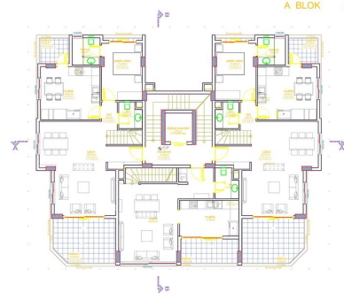
A-D-E BLOK 3. KAT PLANI (+11.40 KOTU)
