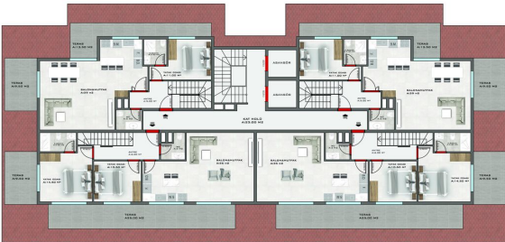
1159/1 KESTEL / A BLOK ÇATI KAT PLANI
