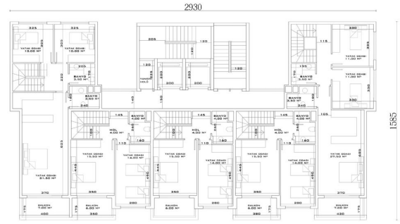
B - C BLOK BAÑÇE DUBLEKS ÜST KAT PLANI
