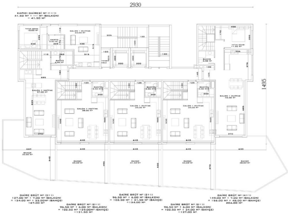
B - C BLOK BAÑÇE DUBLEKS ALT KAT PLANI
