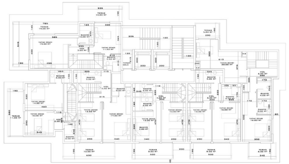
A - D BLOK DUBLEKS ÜST KAT PLANI
