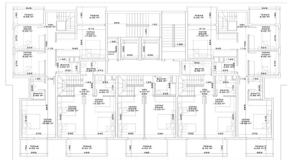
B - C BLOK DUBLEKS ÜST KAT PLANI
