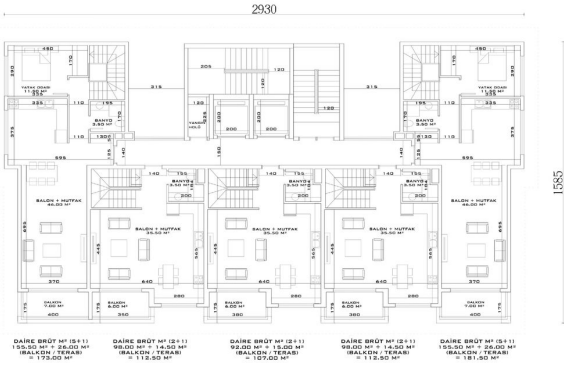
B - C BLOK DUBLEKS ALT KAT PLANI
