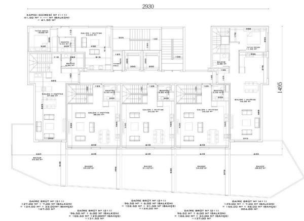
B - C BLOK BANÇE DUBLEKS ALT KAT PLANI
