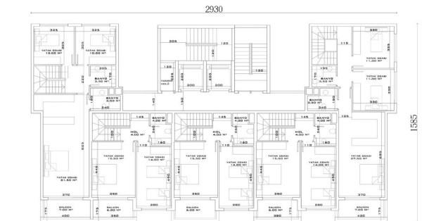
B - C BLOK BANÇE DUBLEKS ÜST KAT PLANI
