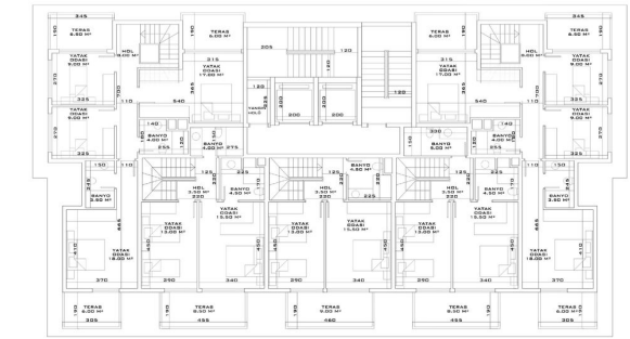
B - C BLOK DUBLEKS ÜST KAT PLANI
