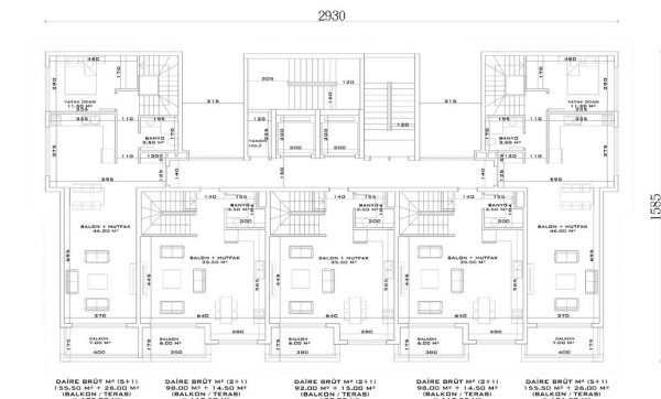
B - C BLOK DUBLEKS ALT KAT PLANI
