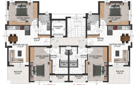
4. KAT PLANI
