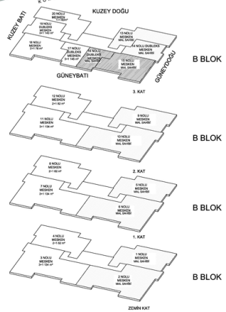
VAZİYET PLANI
