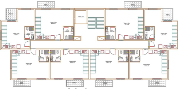
ÜÇÜNCÜ KAT PLANI
