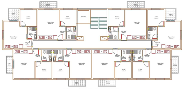
BİR ve İKİNCİ KAT PLANI
