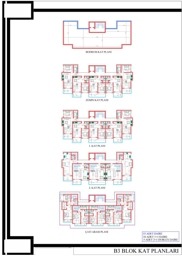
B3 BLOK KAT PLANLARI
