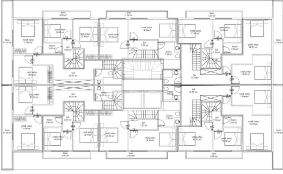
DUBLEKS ÜST KAT
