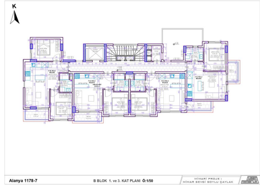
Alanya 1178-7 B BLOK 1. VE 3. KAT PLANI 0:150 MİMARİ PROJE: MİMAR BEVİSİ BOYLU ÇAYLAK
