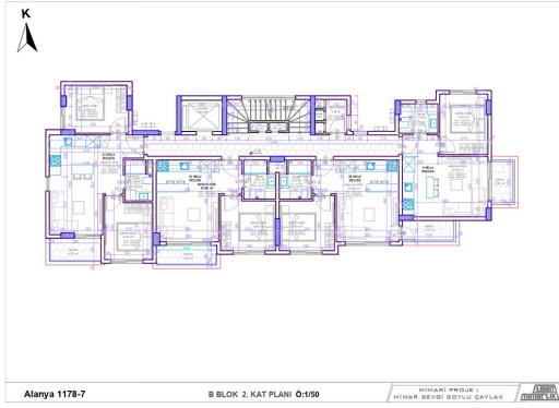
Alanya 1178-7 B BLOK 2. KAT PLANI 0:150 MİMARİ PROJE: MİMAR BEVİSİ BOYLU ÇAYLAK
