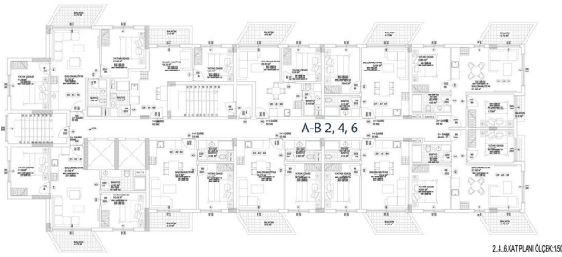
2.4.6KAT PLANI ÖLÇEK 1/50
