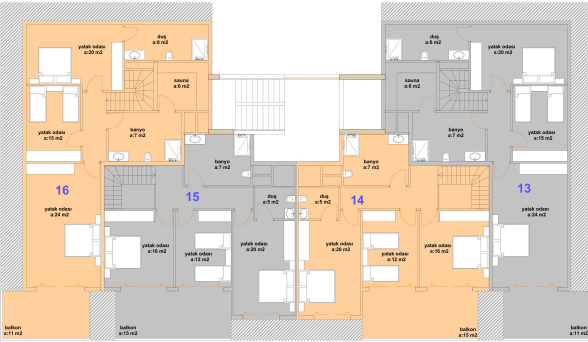
A-B BLOK çatı kat
