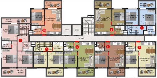
F BLOK / ZEMİN KAT PLANI
