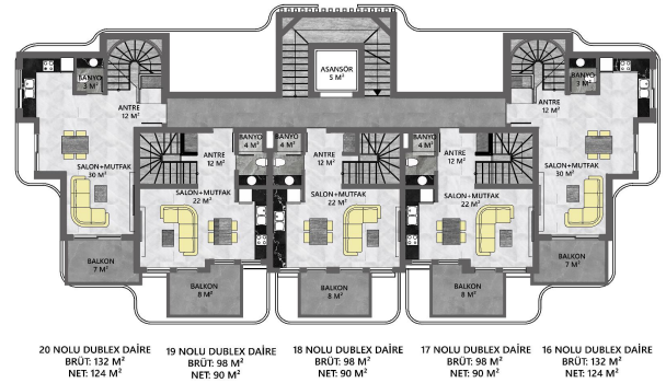
A BLOK 3. KAT PLANI
