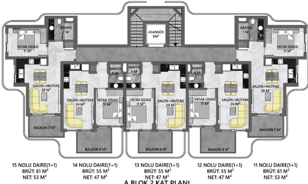
A BLOK 2.KAT PLANI
