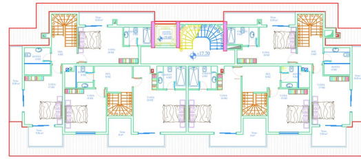
DUBLEX ÜST KAT PLANI
