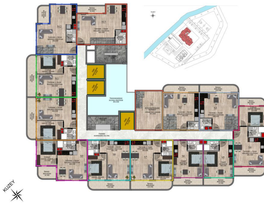
11. KAT PLANI
