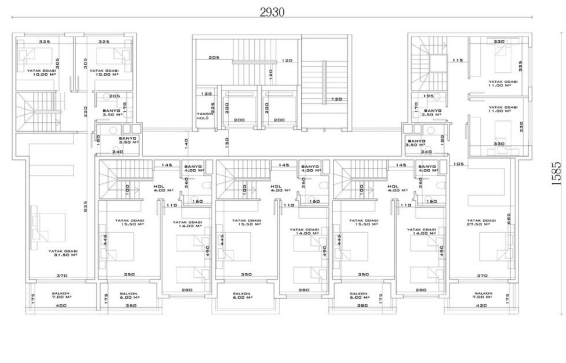
B - C BLOK BAÑÇE DUBLEKS ÜST KAT PLANI
