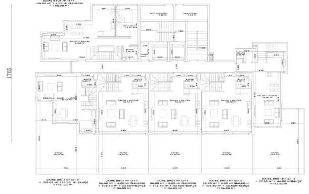
A - D BLOK BAÑÇE DUBLEKS ALT KAT PLANI
