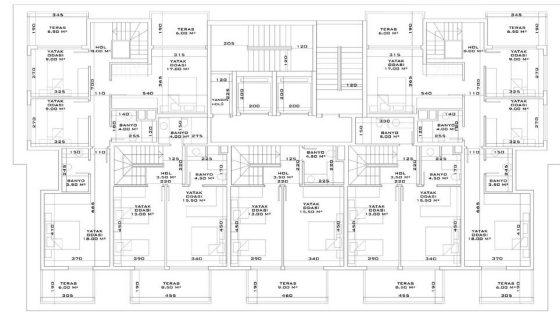
B - C BLOK DUBLEKS ÜST KAT PLANI
