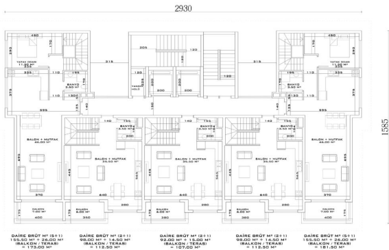
B - C BLOK DUBLEKS ALT KAT PLANI
