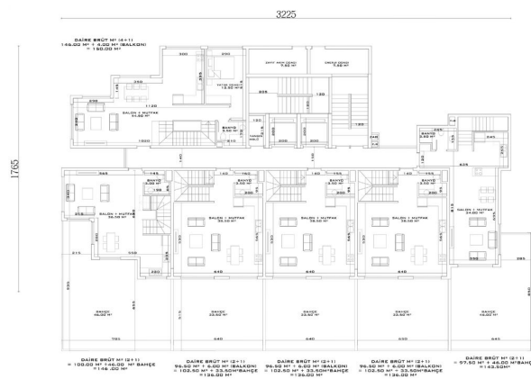
A - D BLOK BAÑÇE DUBLEKS ALT KAT PLANI
