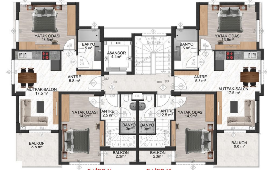
4. KAT PLANI
