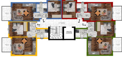
2. KAT PLANI 8 NOLU DAIRE 54 m 2 9 NOLU DAIRE 54 m 2 10 NOLU DAIRE 49 m 2 11 NOLU DAIRE 49 m 2
