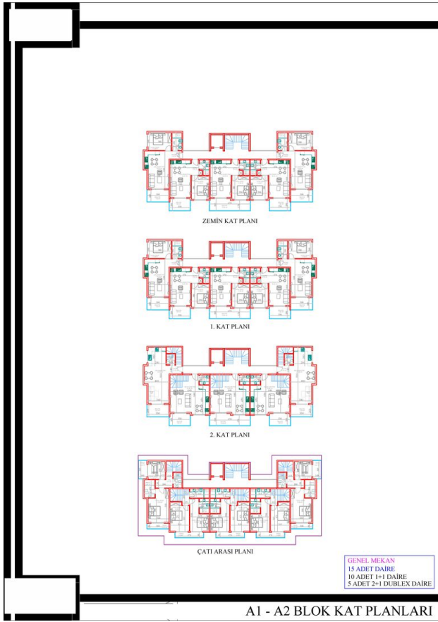
A1 - A2 BLOK KAT PLANLARI
