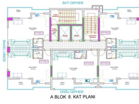
A BLOK 8. KAT PLANI
