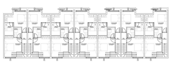
B BLOK ZEMİN KAT PLANI
