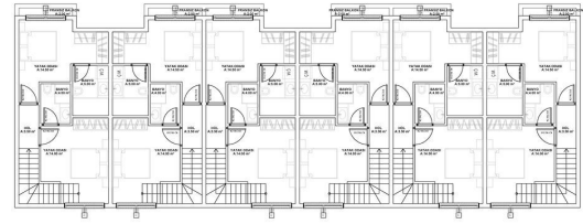
A-C BLOK ZEMİN KAT PLANI
