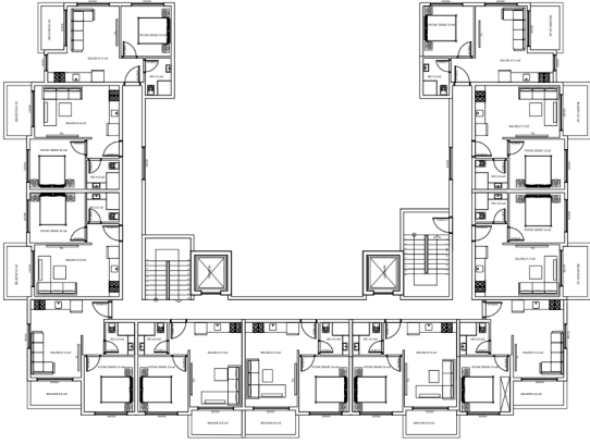
1.2.3.4.5.6.7.8. KAT PLANI
