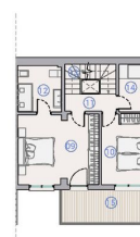
Planta / Floor Intermedia
