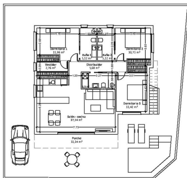
SUP. CONSTRUIDA VIVIENDA - Planta baja 116,58 m 2 - 50% porche 5,57 m 2 VILLA - planta baja Escala 1:100
