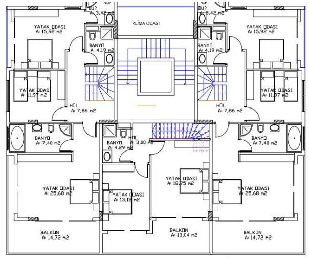
TERS DUBLEKS ÜST KAT PLANI
