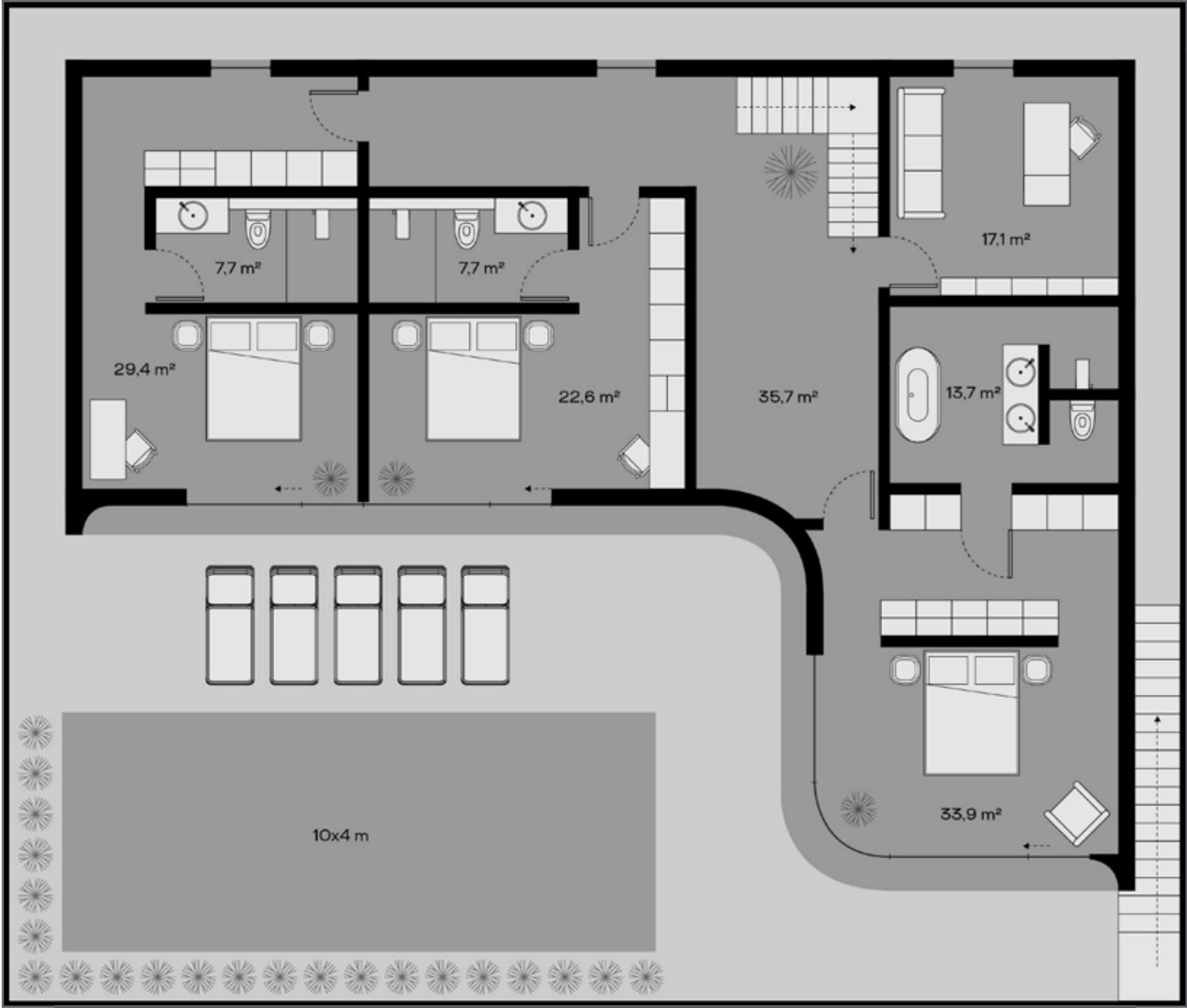
2-ой этаж
