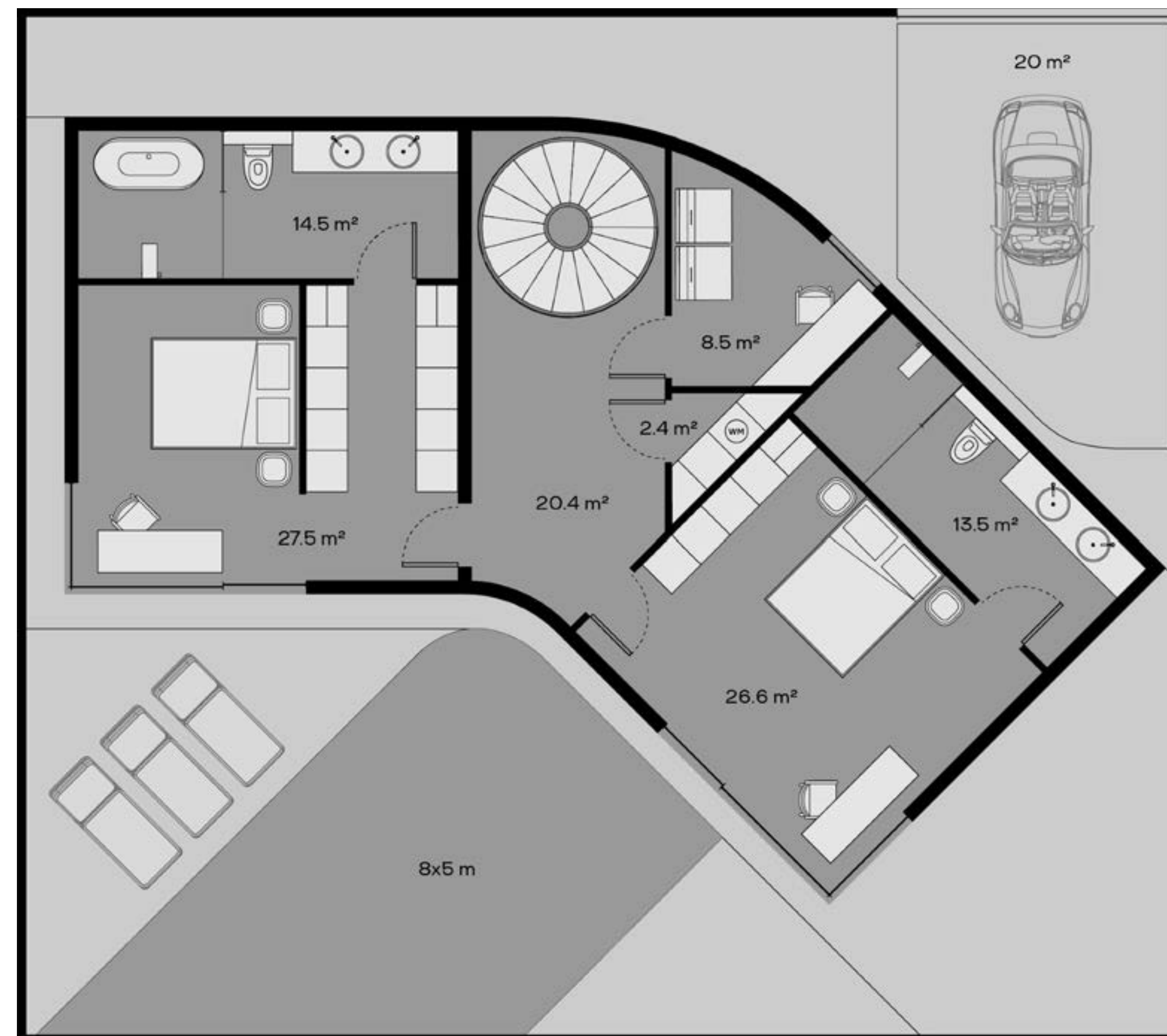
2-ой этаж
