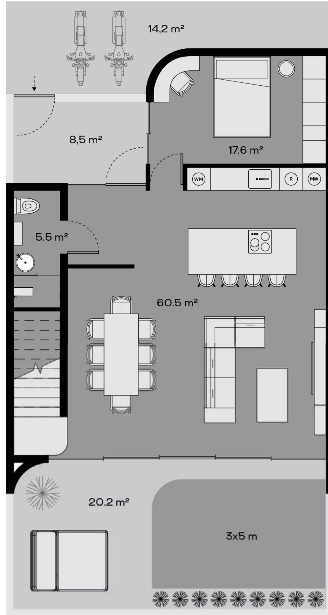
1-ый этаж
