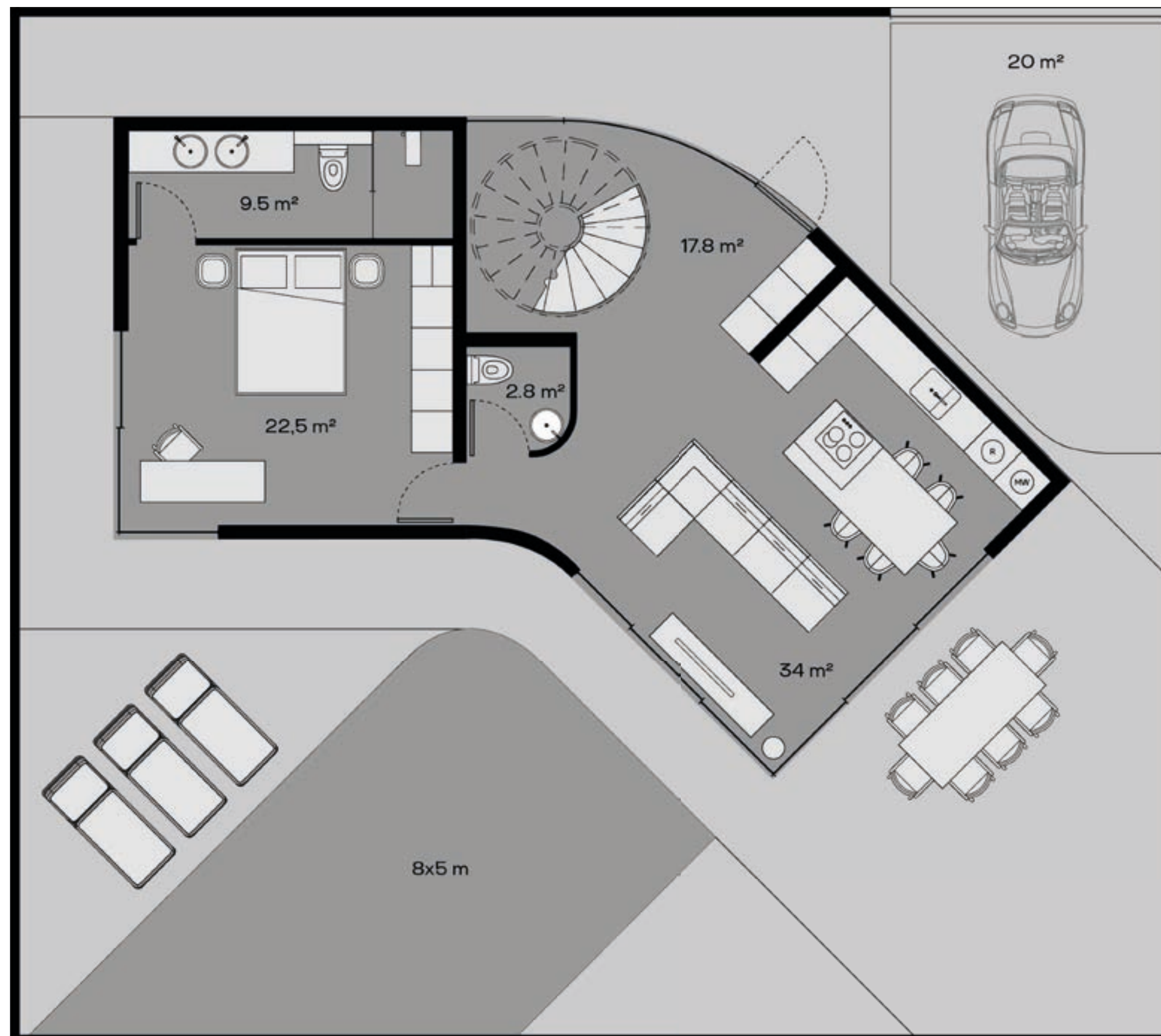
1-ый этаж
