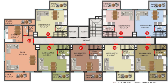
F BLOK / ÜÇÜNCÜ KAT PLANI
