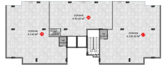
A BLOK ZEMİN KAT PLANI
