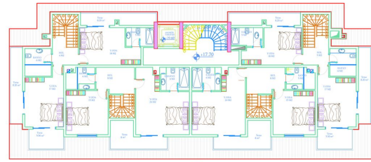
DUBLEX ÜST KAT PLANI
