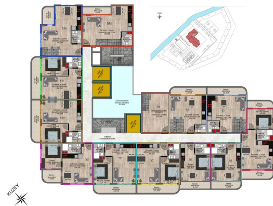
11. KAT PLANI
