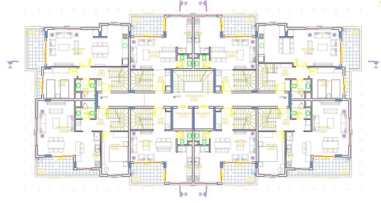
C BLOK 3. KAT PLANI (+11.40 KOTU)
