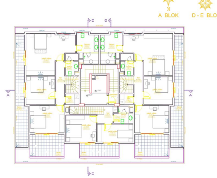
A-D-E BLOK ÇATI ARASI PLANI (+14.70 KOTU)
