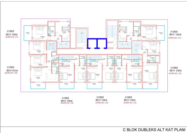
C BLOK DUBLEKS ALT KAT PLANI
