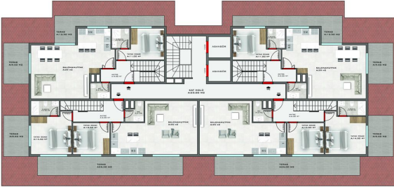
1159/1 KESTEL / C BLOK ÇATI KAT PLANI
