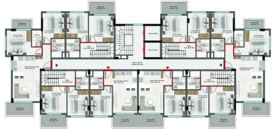
1159/1 KESTEL / C BLOK 3. KAT PLANI
