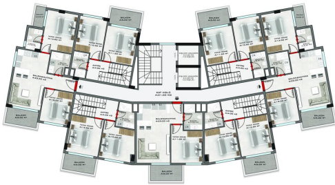
1159/1 KESTEL / B BLOK 3. KAT PLANI
