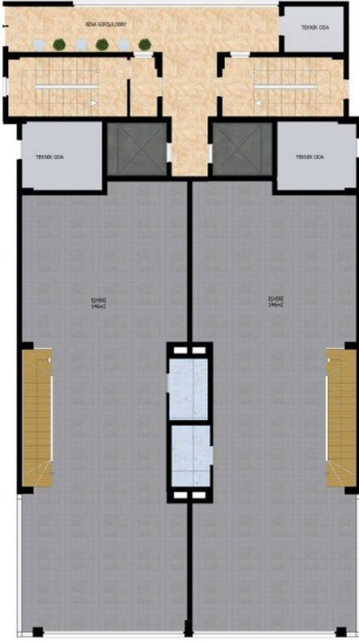
ZEMİN KAT PLANI
