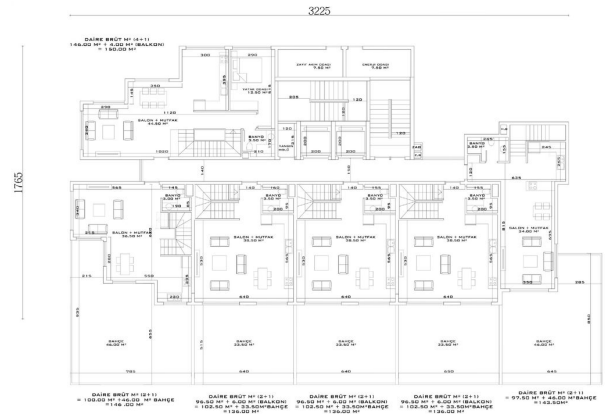
A - D BLOK BAĞÇE DUBLEKS ALT KAT PLANI
