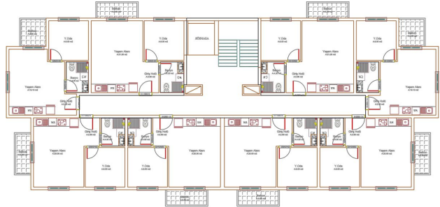
BİR ve İKİNCİ KAT PLANI
