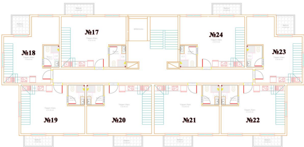
ÜÇÜNCÜ KAT PLANI
