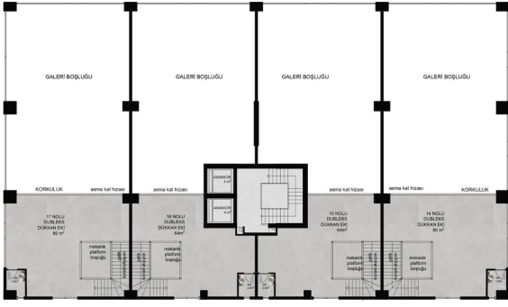
B BLOK / ASMA KAT PLANI
