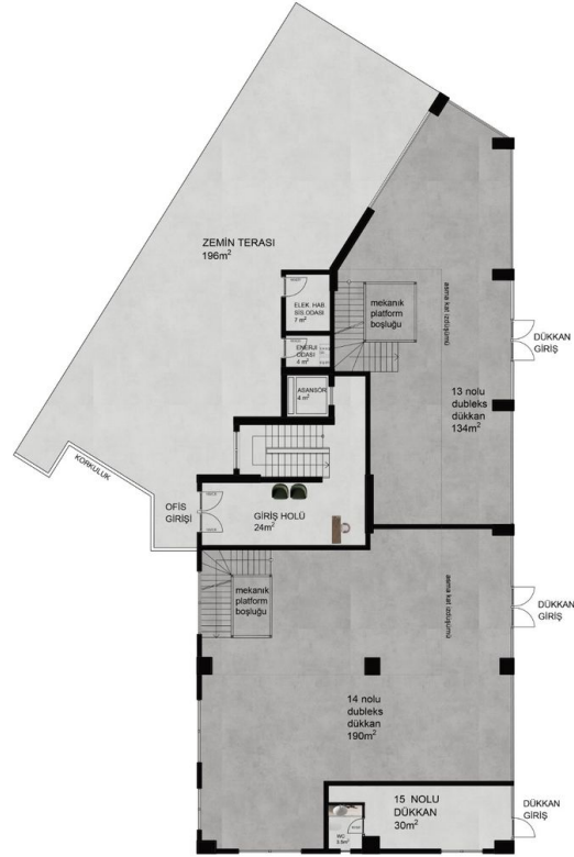
C BLOK /ZEMİN KAT PLANI
