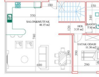
ZEMİN KAT PLANI
