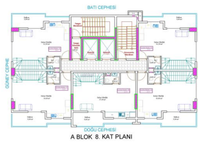
DOĞU CEPHESI A BLOK 8. KAT PLANI
